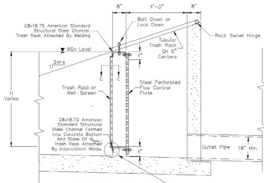
Section A-A
